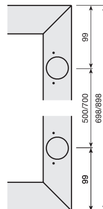
Montage der Türen mit Leisten
