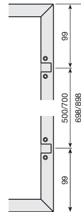
Montage Türen mit Leisten
