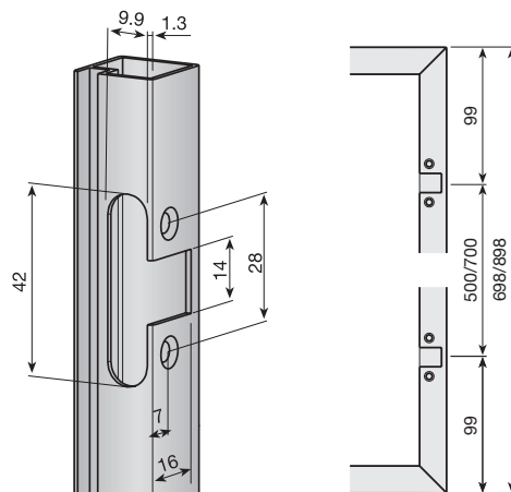
Bearbeitung und Anordnung der Scharniere
