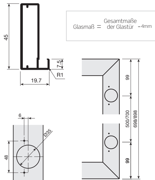
Bearbeitung und Anordnung der Scharniere
