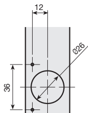
Bearbeitung Profile 35x20
