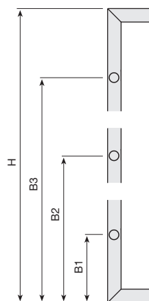
Bearbeitung für 3 Scharniere
