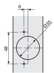
Bearbeitung und Anordnung der Scharniere
