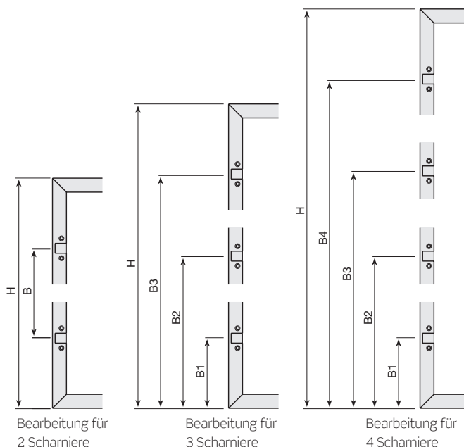
Bearbeitung und Anordnung der Scharniere
