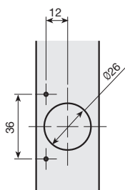
Bearbeitung und Anordnung der Scharniere
