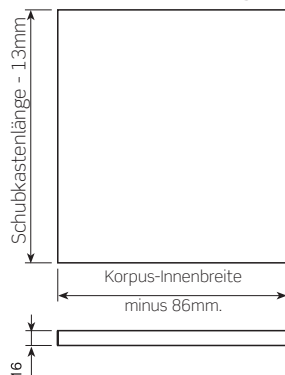
Bodenberechnung
