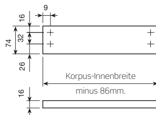
Rückwandberechnung
