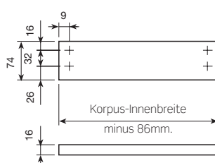
Rückwandberechnung
