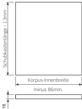
Bodenberechnung
