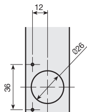
Usinage Profils 35x20
