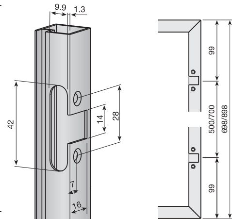
Usinage et positionnement des charnières.
