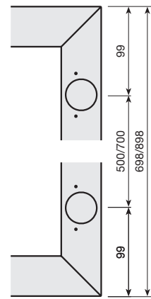
Assemblage des portes avec traverses
