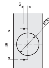
Usinage et positionnement des charnières
