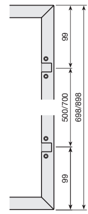
Usinage et positionnement des charnières
