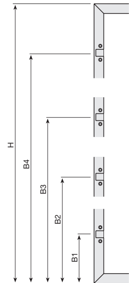
Usinage pour 4 Charnières
