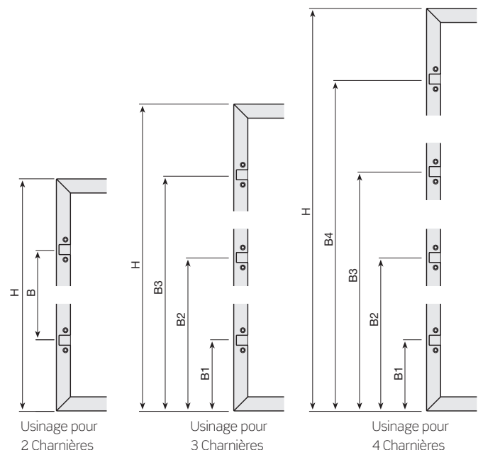
Usinage et positionnement des charnières.
