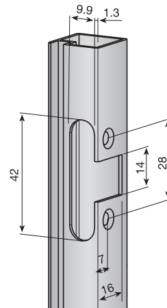
Usinage et positionnement des charnières
