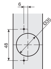
Usinage Profils 45x20
