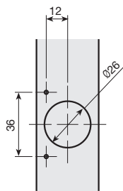
Usinage et positionnement des charnières
