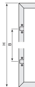
Usinage pour 2 Charnières
