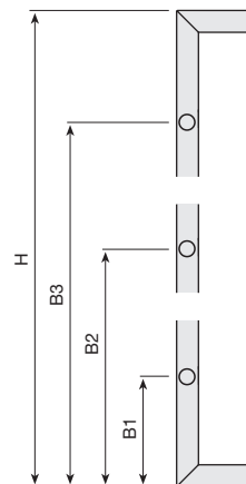
Usinage pour 3 Charnières
