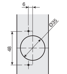
Usinage et positionnement des charnières
